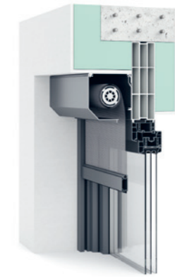
VS-Z 45°. Rollgeformte Blenden und stranggepresste Revisionsblende, Einbausituation WDVS.
