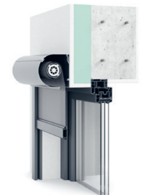
VS-Z rund. Rollgeformte Blenden und stranggepresste Revisionsblende, Einbausituation WDVS.
